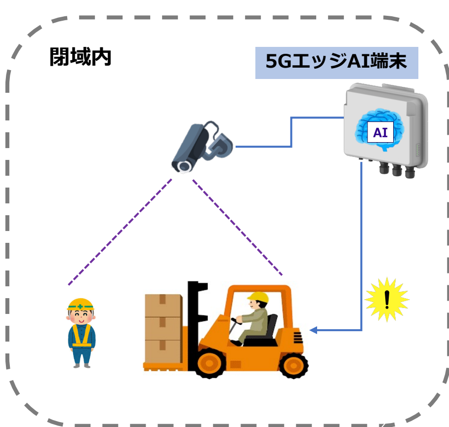
case 1: フォークリフトの接近検知 →フォークリフトと作業員の過度な接近を検知し、フォークリフトを自動停止させる信号を送信します
