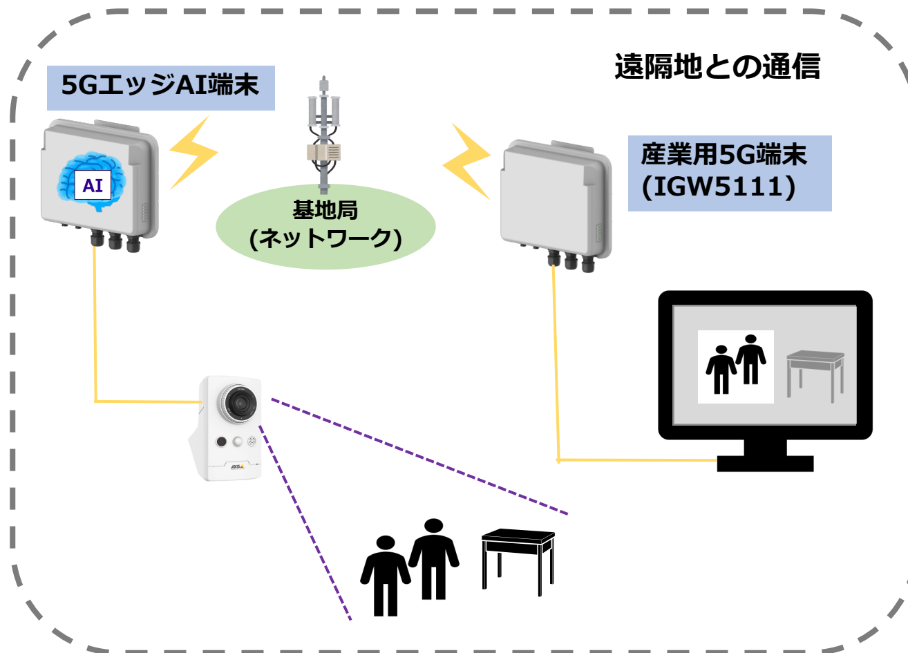
case 2: 施設内の対象物の高画質映像伝送 →AI画像処理に基づいた映像圧縮技術により 注目したい対象物(人・機械など)のみを高画質で伝送します
